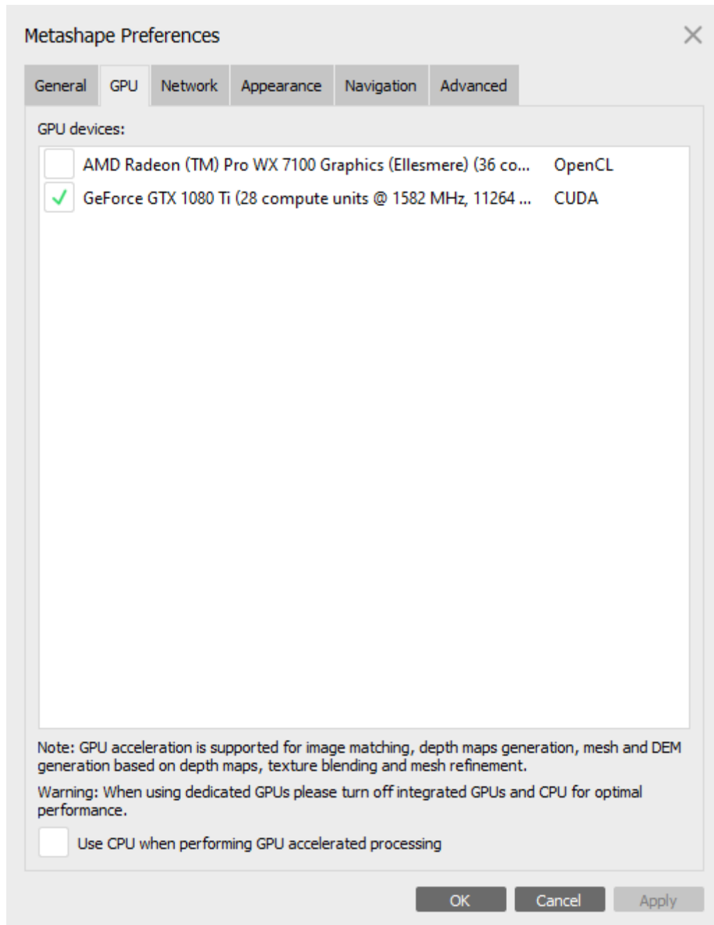
GPU tab
