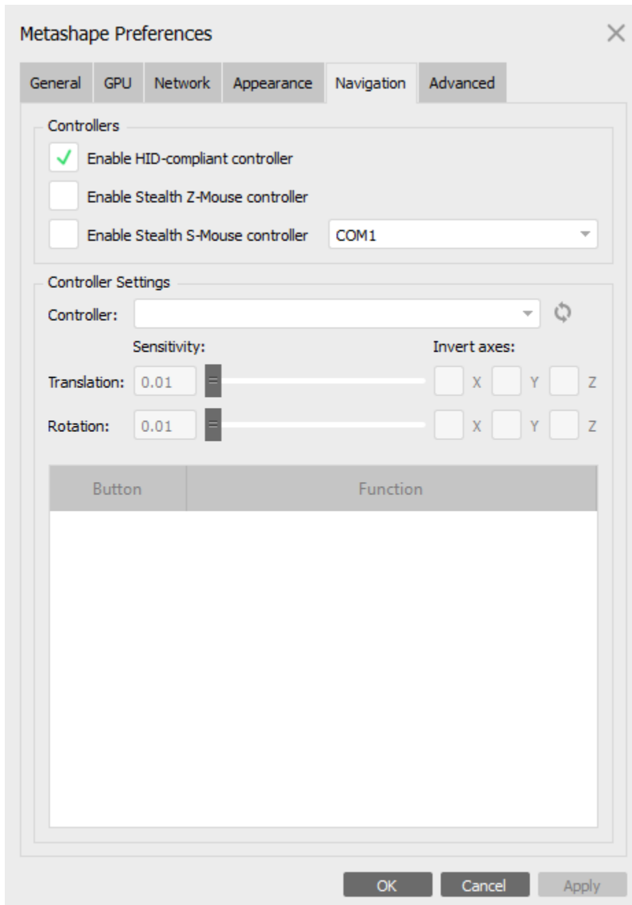
Navigation tab
